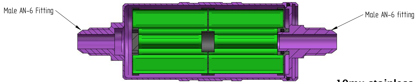
SECTION A-A
